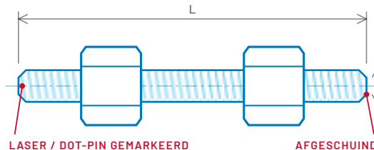
STUD BOLT + 2 ZESKANTMOEREN
